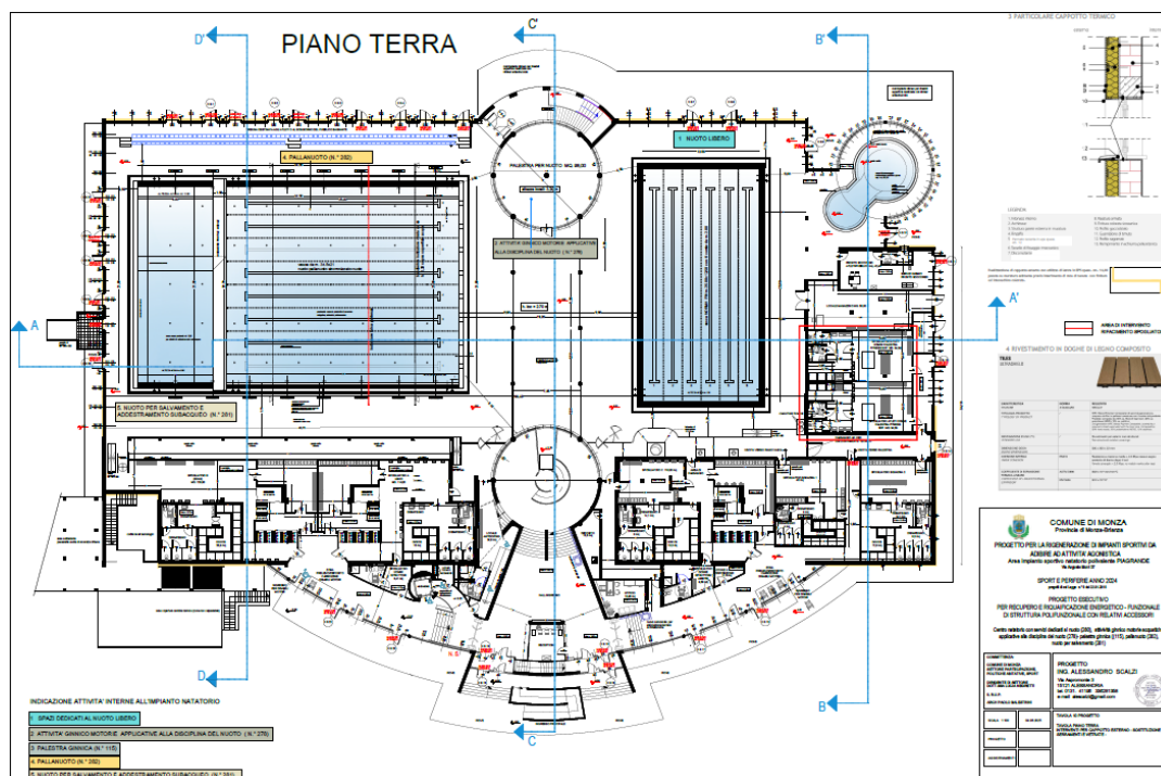
Planimetrie di progetto
