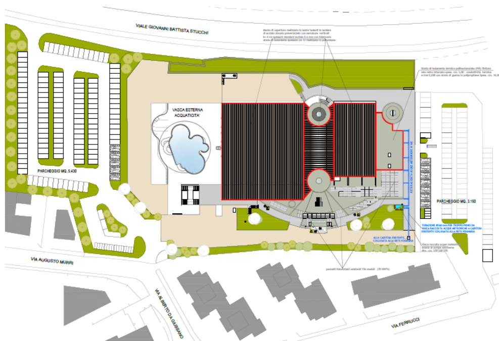
Planimetria Generale - interventi di copertura
