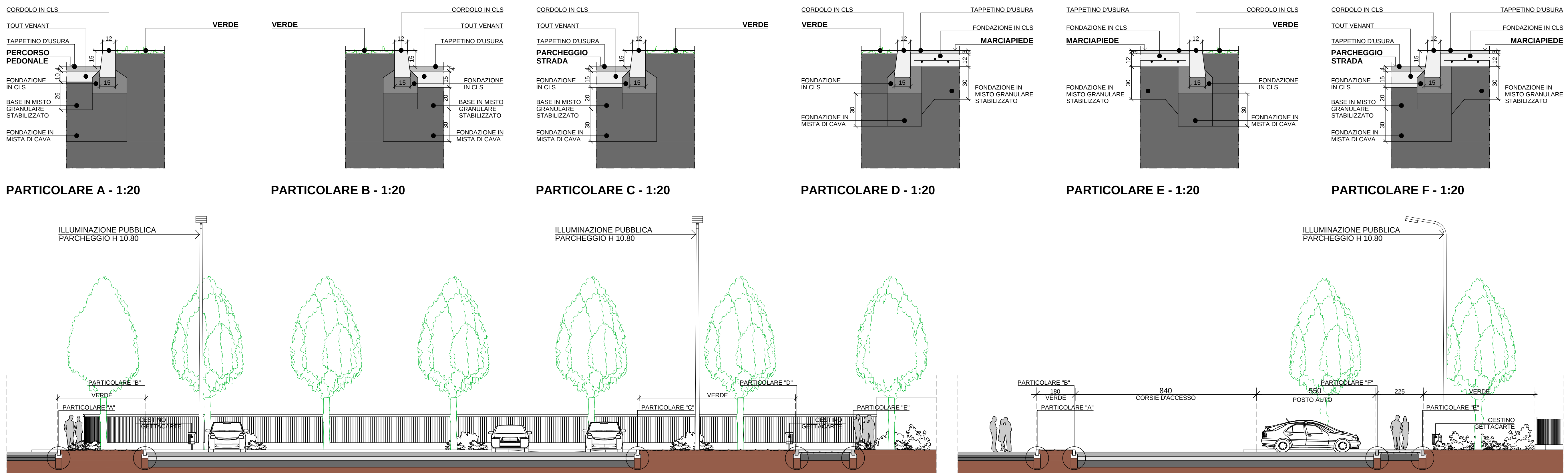
SEZIONE 1-1 SCALA 1:100
