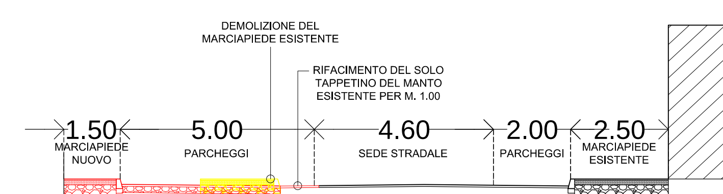
SEZIONE B-B VIA QUARNARO
