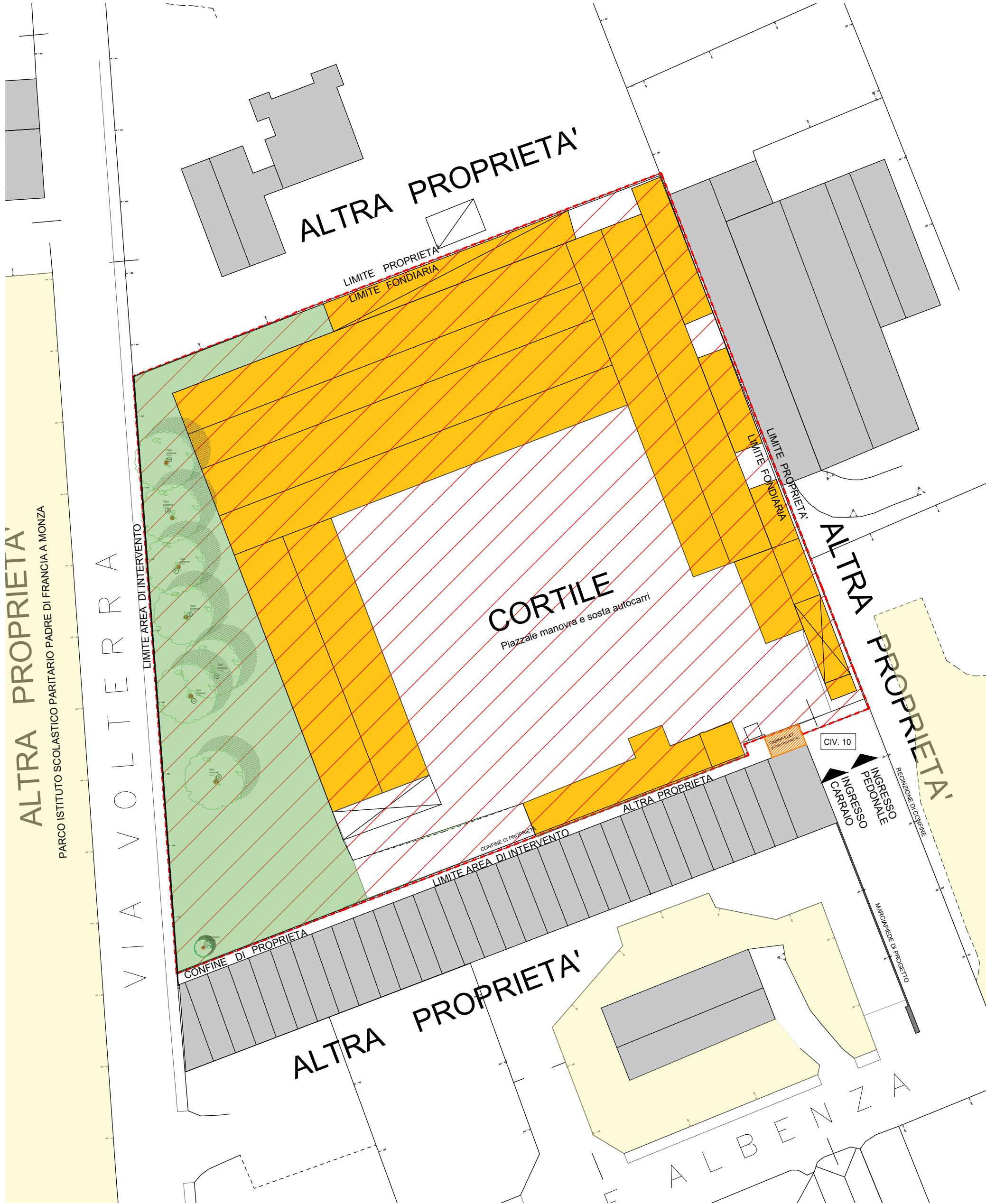
K-PLAN STATO DI FATTO
