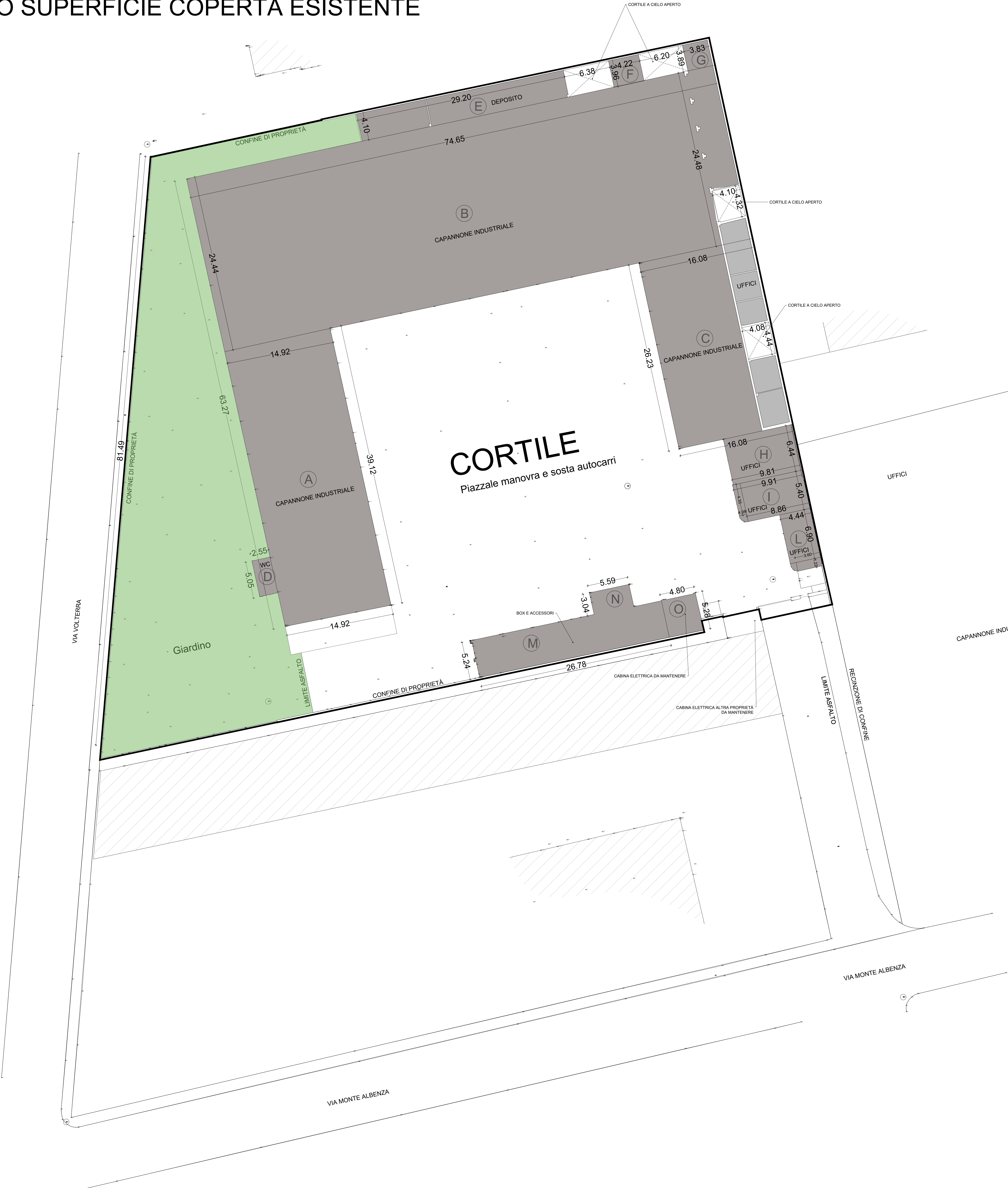
PLANIMETRIA GENERALE SCALA 1:200
