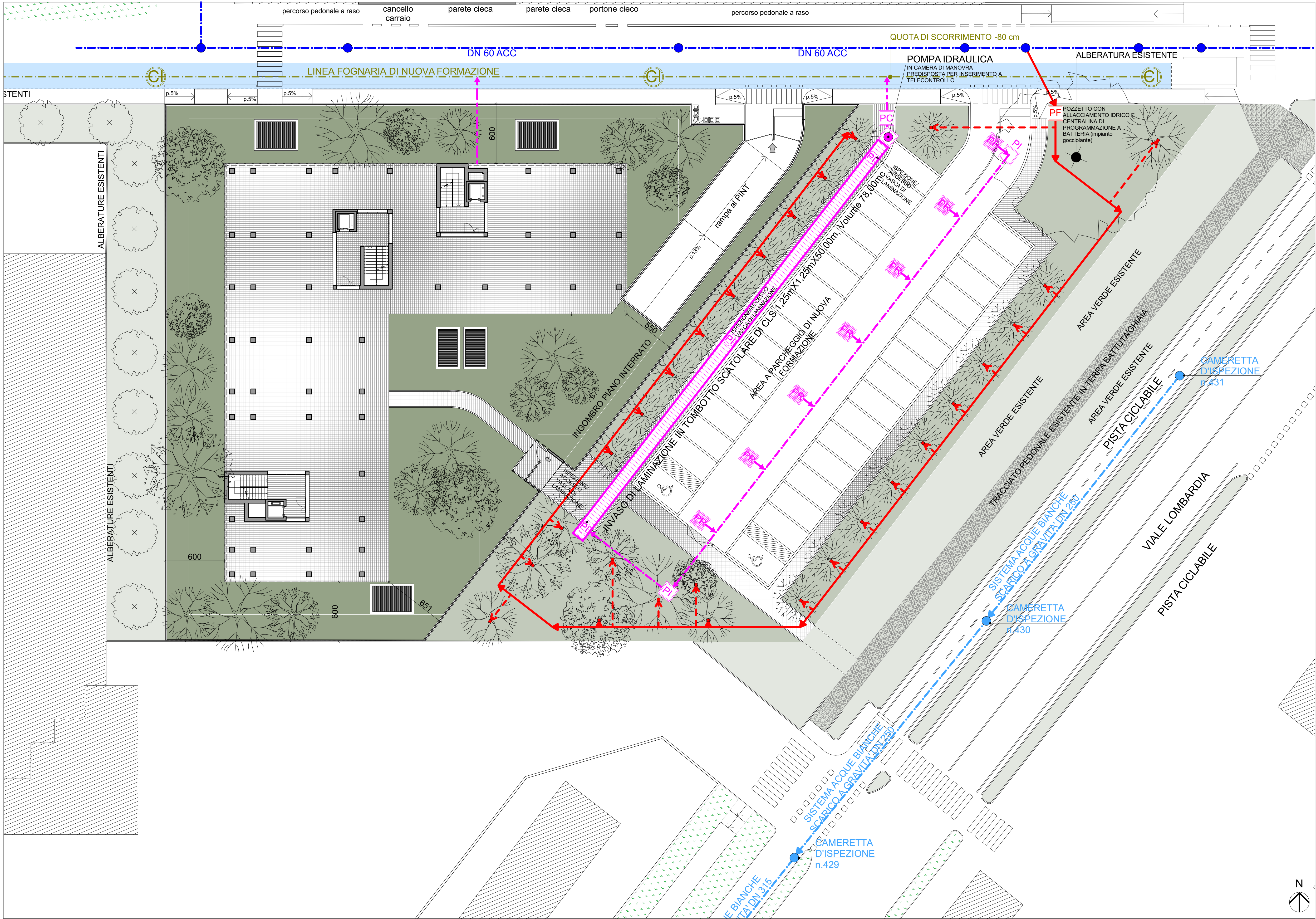
SCHEMA FOGNATURA E IMPIANTO IDRICO - STATO DI PROGETTO - scala 1:200
